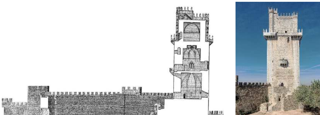
Figuras 019 e 020 | Corte Longitudinal e alçado nascente da torre de menagem de Beja
