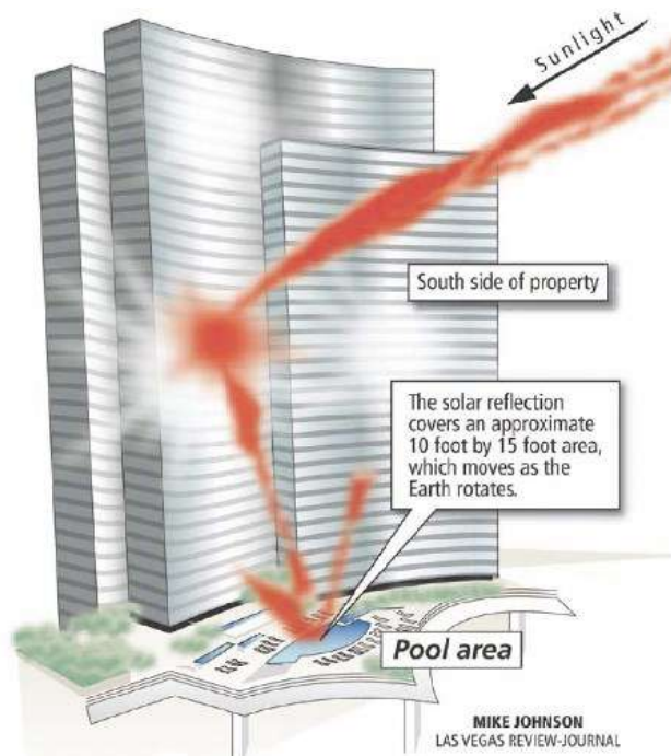
Figuras 114 e 115 | Edifício "Vdara Hotel" e esquema do problema
