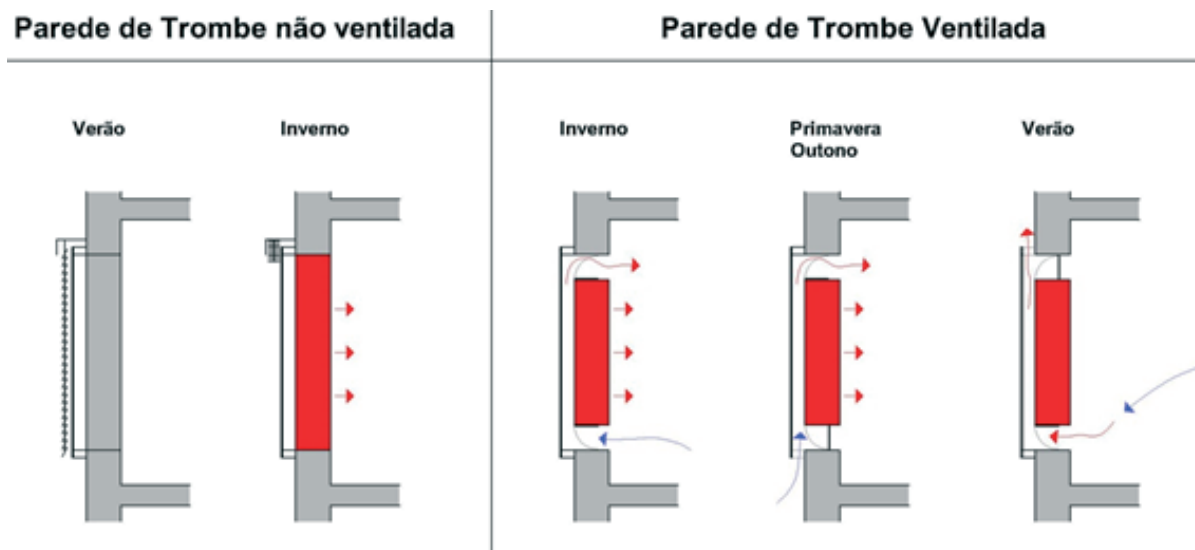
Figura 6 - Parede de Trombe ventilada e não ventilada.
