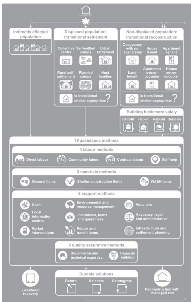
Gráfico 6 - Diagrama de fluxos para intervenção em situações de emergência.
