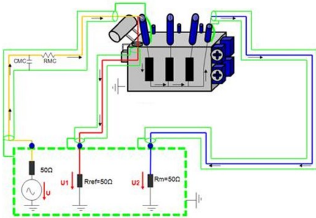
Analisador FRA
