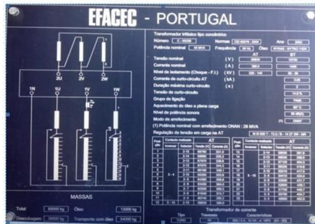
Figura 47: Chapa de características para comparação de resultados [EDP].
