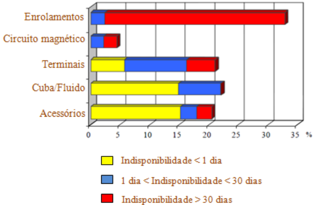
Figura 31: Indisponibilidade do transformador associado a cada tipo de avaria [40].
